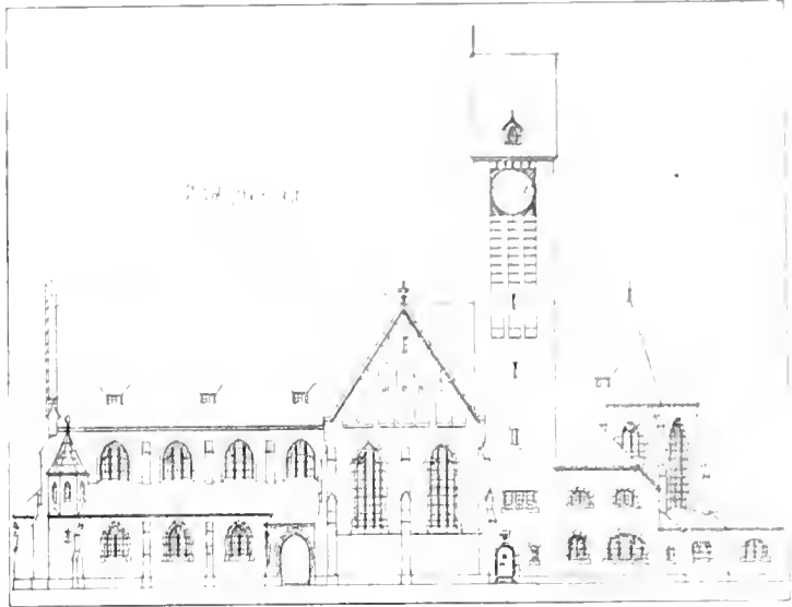
MOTTO QUERSCHNITT SÜDLICHE AUSSENANSICHT Nr. 16, Text S. VII, 22, Nr. 15 und 17
